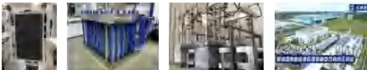
大面积膜电极、大气量电解槽、国内首套兆瓦级系统及示范应用
