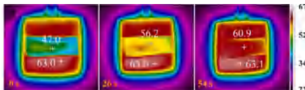
热管理性能
